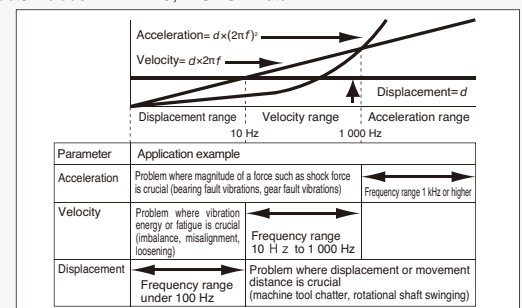
Vibration parameter
